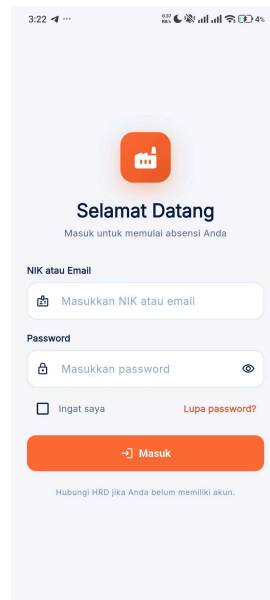
Gambar 4.1. Halaman login
